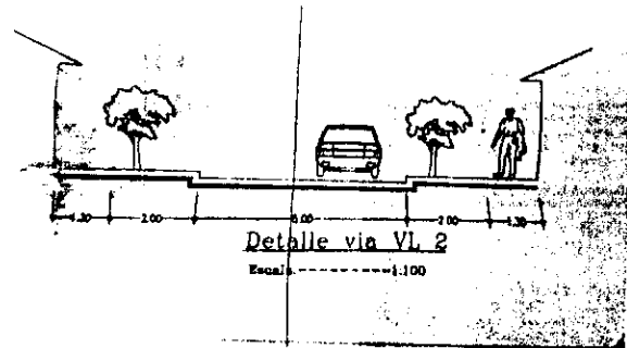
Foto No. 3 y 4. Planteamiento urbanístico para el barrio Samaria aprobado en el año 2003. VL 2 Andén 1,30 m, zona verde 2,00, calzada 5,00 m, zona verde 2,00 m y andén 1,30 m. El perfil vial se encuentra modificado en sitio ya que primero es la zona verde y luego el andén.
